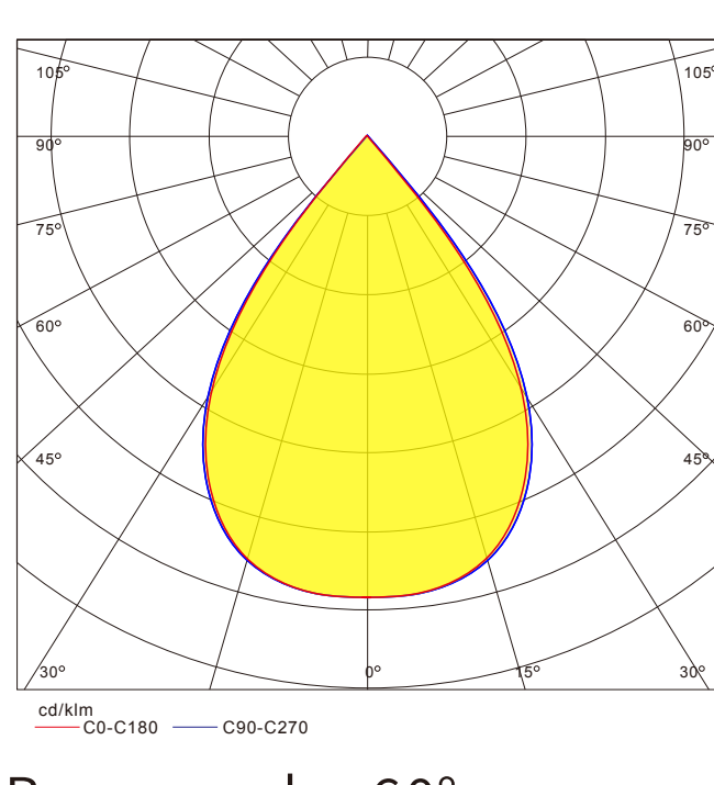
Beam angle: 60°
