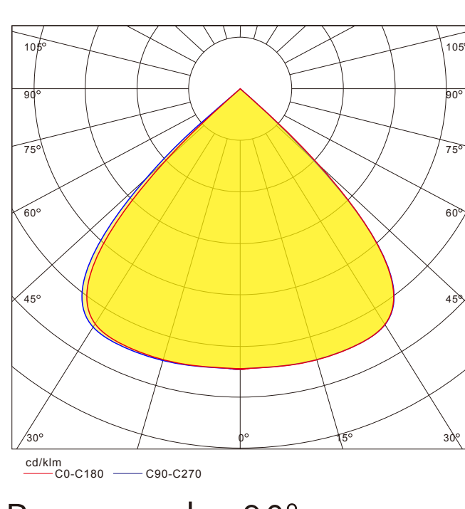
Beam angle: 90°
